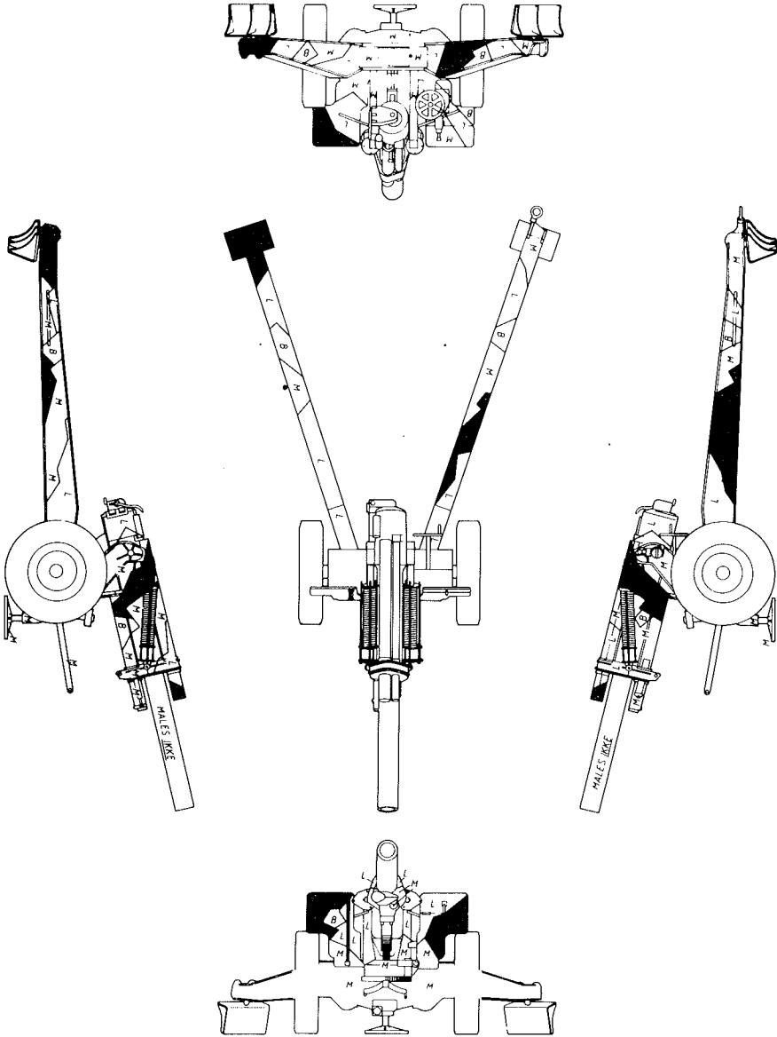
155 mm HAUBITS M 144
